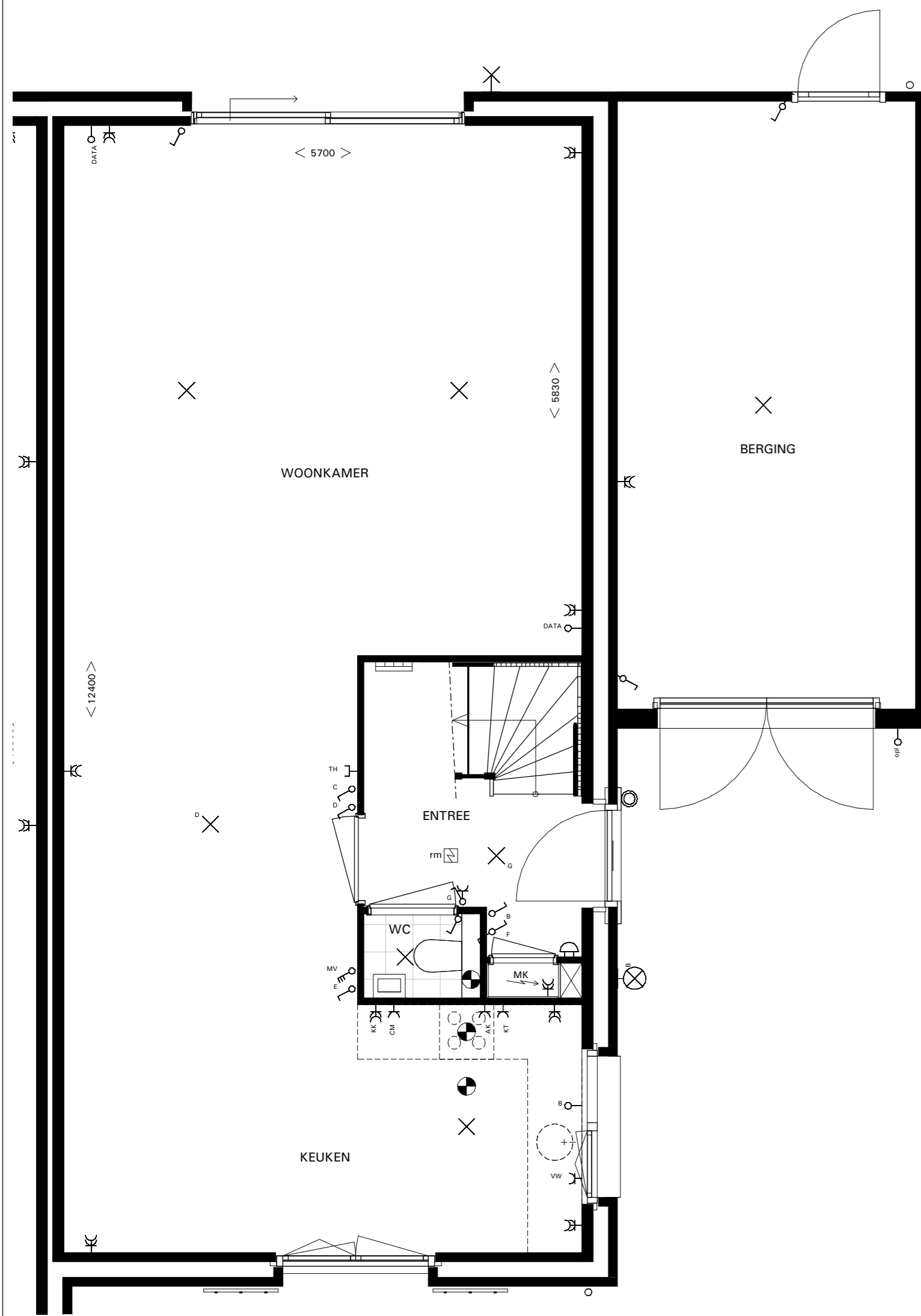
BEGANE GROND
