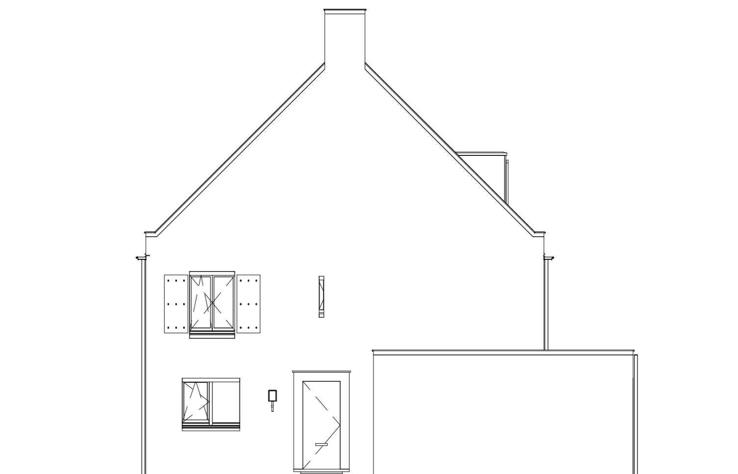
RECHTER ZIJGEVEL
